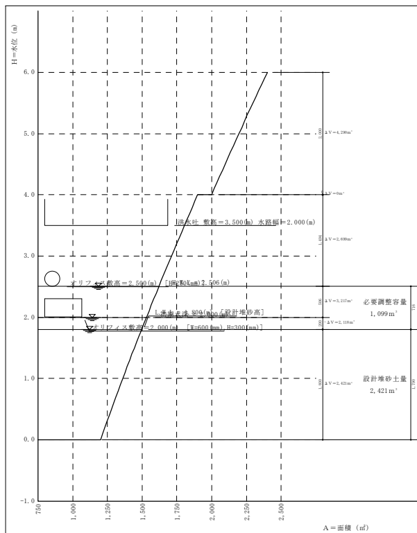
H-A 曲線
